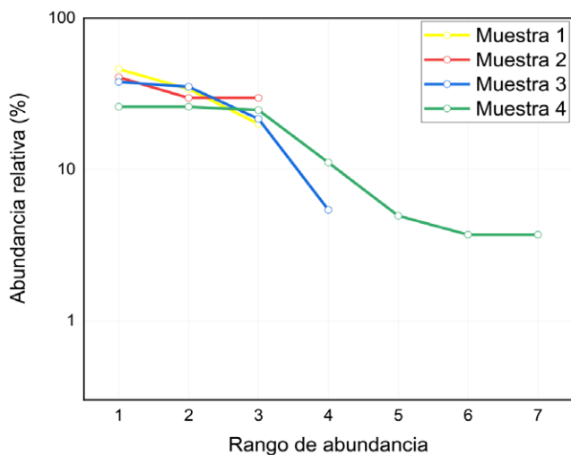
Figura 4. Diagrama rango-abundancia de las especies distribuidas en las muestras colectadas del sitio. El rango de abundancia varía desde el organismo más abundante hasta el de menor abundancia (eje x), y la abundancia relativa se expresa en un eje \log_{10} . La aplicación de curvas de rango-abundancia se encuentran menos limitadas por los cambios taxonómicos que otros métodos cuantitativos, lo que permite evaluar la respuesta ecológica del conjunto de diferentes organismos ante el estrés ambiental en el ecosistema.
