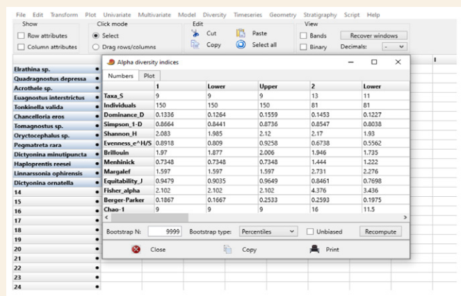
Figura 7. Por medio de la opción "índices de diversidad" es posible conocer los distintos valores para los índices ecológicos anteriormente descritos tales como Índice de Dominancia de Simpson (1949), Índice de Equitatividad de Simpson (1949), Índice de Diversidad de Shannon (1949), Índice de Diversidad de Menhinick (1964), Índice de Riqueza Total de Chao (2005).
