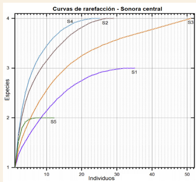
Figura 5. Curvas de rarefacción basadas en el registro y abundancia de organismos fósiles del Cámbrico, distribuidos en una unidad litoestratigráfica del centro del estado de Sonora, México (Tomado de Cuen-Romero et al., 2019) [34]. En este diagrama se observan cinco curvas las cuales corresponden a cinco estratos dentro de la unidad rocosa, y muestra la relación entre individuos y especies de cada estrato. Los círculos indican las especies o individuos que se cuantificaron.
