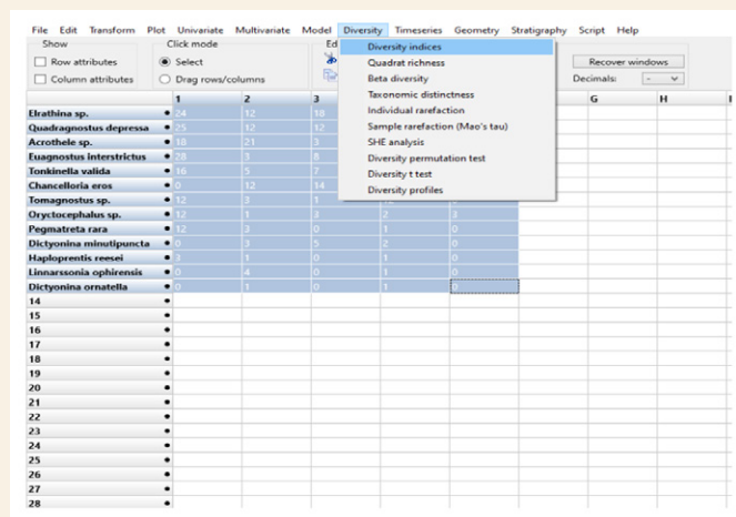
Figura 6. El uso del software 3.x ® determina diversos análisis estadísticos. La aplicación permite determinar índices de diversidad y rarefacciones individuales, así como otros estimadores para la diversidad Beta, distinción taxonómica, prueba de permutación de diversidad, prueba de t de diversidad, entre otros.
