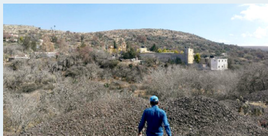
Figura 2. Muestra "de mano" (izquierda). Depósito de escorias muestreados en Monte Caldera (derecha).
