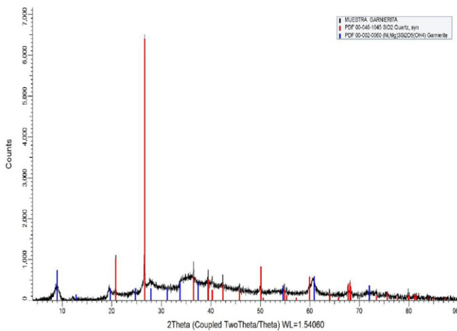
Figura 3. Difractograma de la muestra RD-18-02. Se logran identificar 2 minerales: garnierita y cuarzo. Los picos de intensidad en la señal de conteo para el cuarzo están en un ángulo de difracción ( 2\theta ) de 20.9, 26.5, 37.4, 39.1, 50.1, y 60.9, y algunos otros picos de menor intensidad. Nótese que la señal del cuarzo es máxima en 26.5. Para el caso de la garnierita, los picos en 2\theta , están en 9.0, 19.4, 24.8, 27.9, 31.2, 33.8, 37.4, 54.6, 60.9 y 72.0. Los cuales son consistente con el reporte PDF que identifica positivamente a la garnierita.
