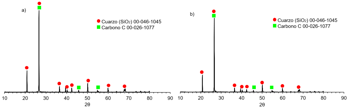
Figura 2. Patrones de difracción para las muestras a) 100 y b) +100, después de la eliminación de carbonato de calcio.
