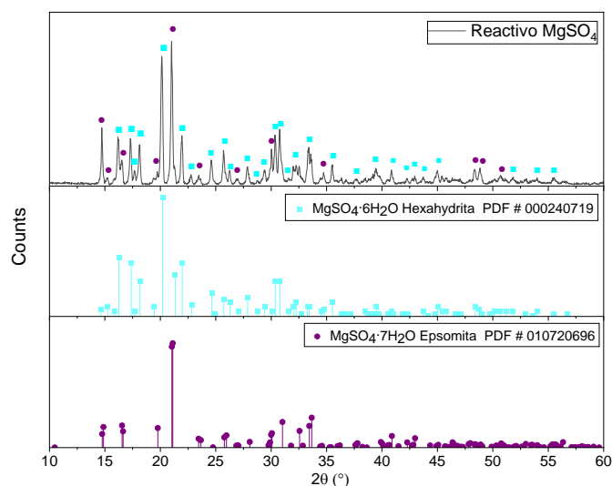
Figura 3. Espectros de difracción de rayos X (DRX) del reactivo de \text{MgSO}_4 \cdot 7\text{H}_2\text{O} .
