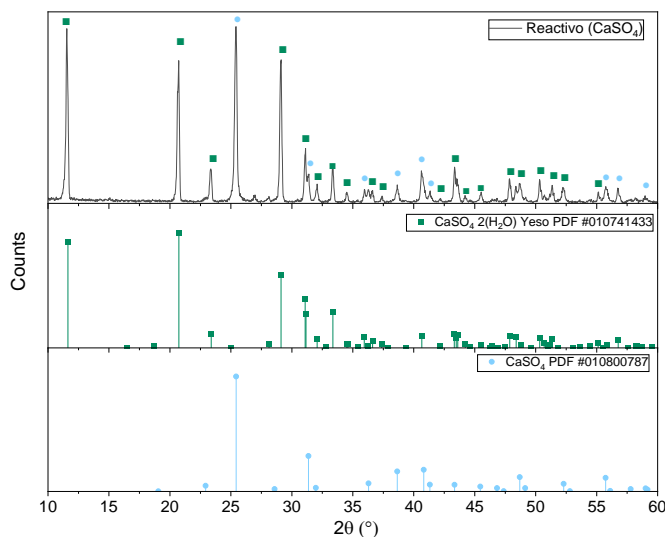
Figura 2. Espectros de difracción de rayos X (DRX) del reactivo de \text{CaSO}_4 \cdot 2\text{H}_2\text{O} .
