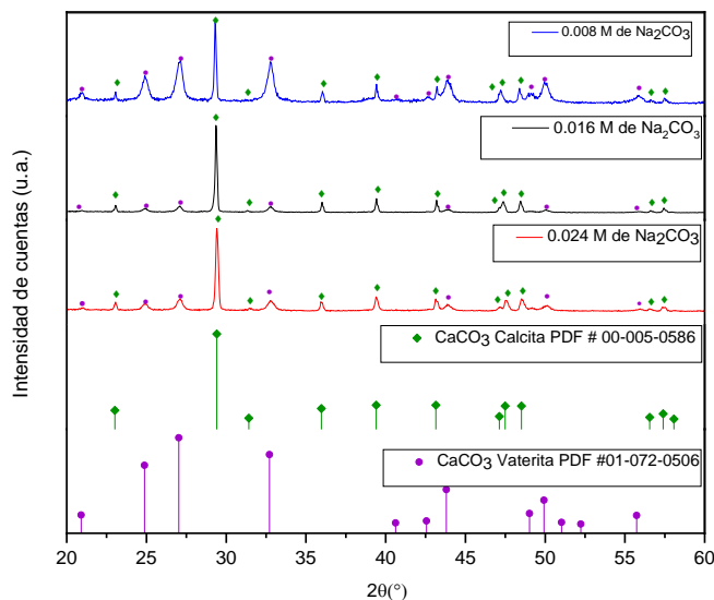
Figura 4. Espectros de difracción de rayos X (DRX) de los sólidos obtenidos de la precipitación de \text{CaCO}_3 en solución mediante la adición de carbonato de sodio (experimentos 10,11 y 12, respectivamente).
