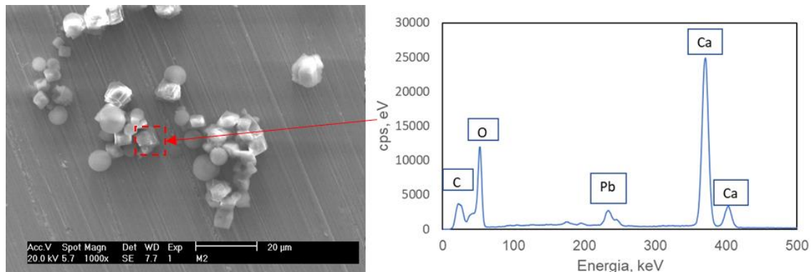
Figura 5. Micrografías MEB y análisis EDS de la interacción superficial entre galena y el calcio precipitado mediante la adición de carbonato de sodio.
