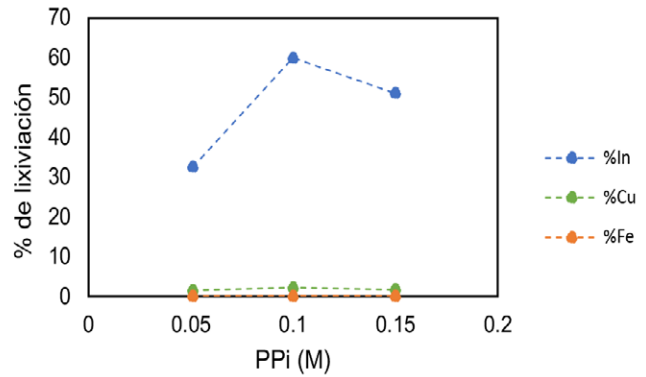
Figura 7. Efecto de la concentración de P_2O_7^{4-} (PPI) en la lixiviación de In, Fe, y Cu.
