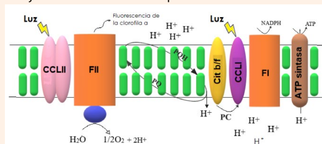
Figura 1. Esquema simplificado del proceso de transporte de electrones que sucede en la membrana tilacoidal de las plantas. FII: Fotosistema II, CCLII: Complejo Cosechador de Luz II, Cit b/f: Citocromo del tipo b y f, FI: Fotosistema I, CCLI: Complejo Cosechador de Luz I, PC: Plastocianina, PQ: Plastoquinona, ATP: Adenosin Trifosfato, NADP: Nicotinamida Adenina Dinucleótido Fosfato (P). La adición del ión H^+ simboliza la reducción de las moléculas. Modificado de Baker y Rosenqvist [11].
